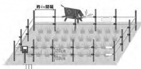
設置イメージ図【イノシシ対策用】
